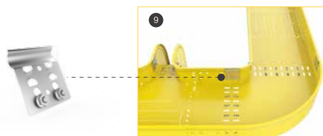
侧面连接板：与各部件连接更牢固，适合独立吊装承重要求。
